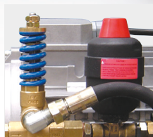
Valvola di regolazione e accumulatore di pressione
